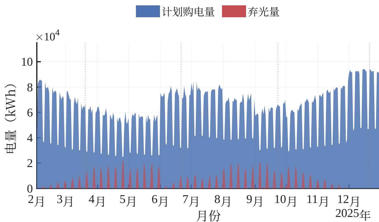
全年逐日购电量与弃光量
